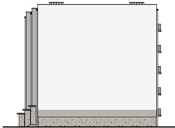
ELEWACJA ZACHODNIA
